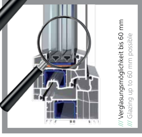
/// 3 Dichtungsebenen /// 3 sealing levels
