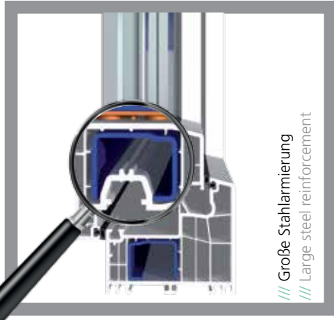
/// Großzügige Falztiefe /// Generous rebate depth
